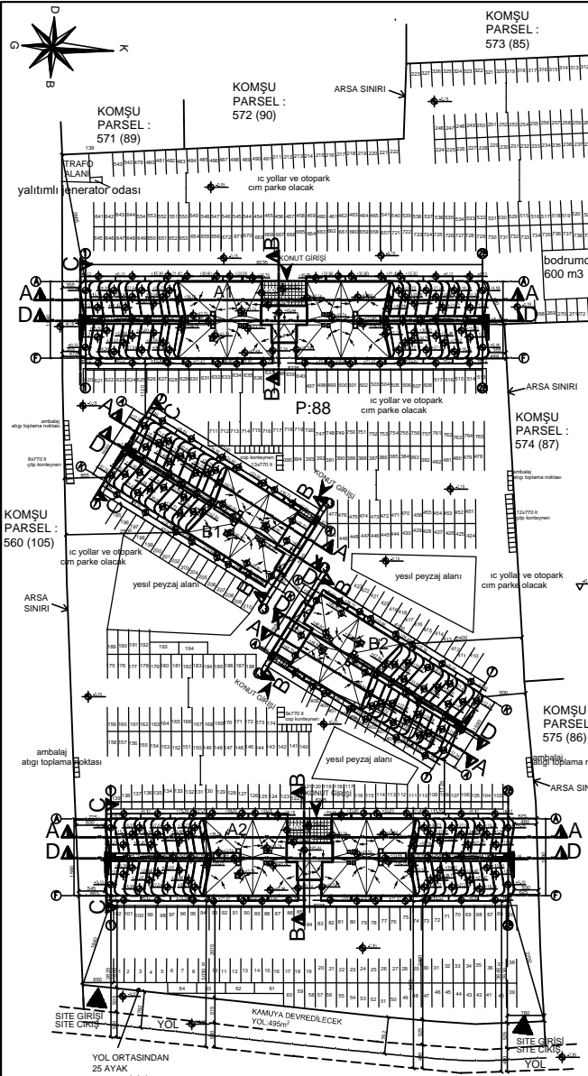
VAZİYET PLANI Ölçek: 1/500
