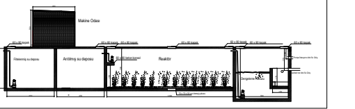
Arıtma A-A Kesiti
