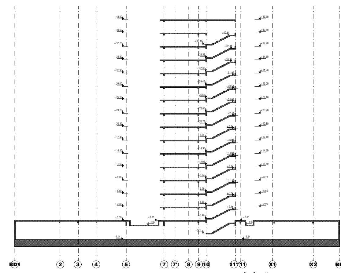
AA KESİTİ ÖLÇEK: 1/500
