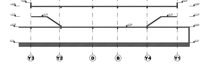
AA KESİTİ ÖLÇEK 1/500
