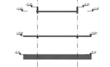
BB KESİTİ ÖLÇEK 1/500
