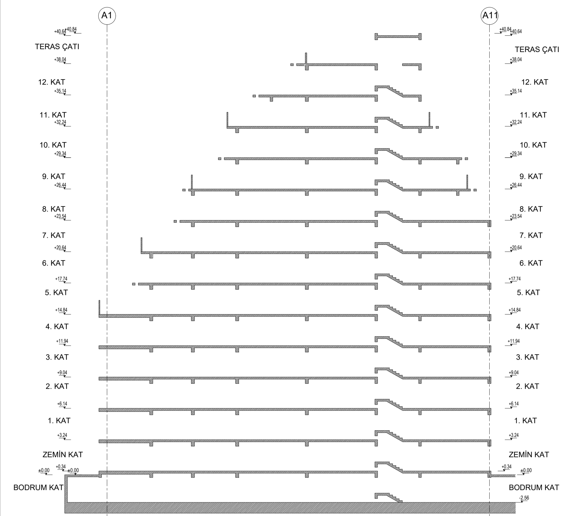
TİP A BLOK 1 AA KESİTİ Ö:1/200
