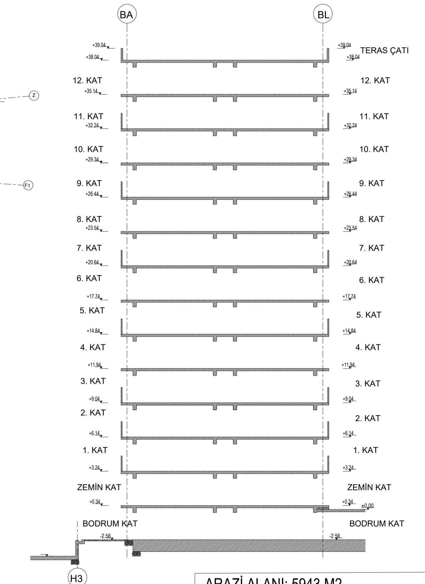
TİP A BLOK 2 DD KESİTİ Ö:1/200
