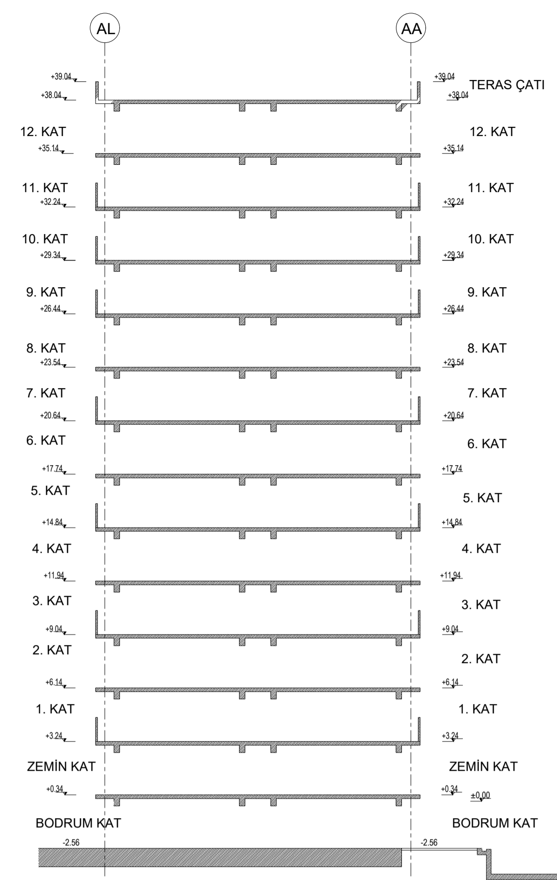
TİP A BLOK 1 BB KESİTİ Ö:1/200
