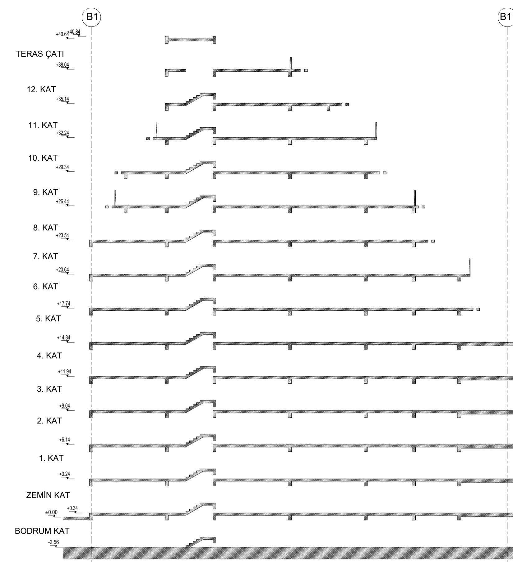
TİP A BLOK 2 AA KESİTİ Ö:1/200
